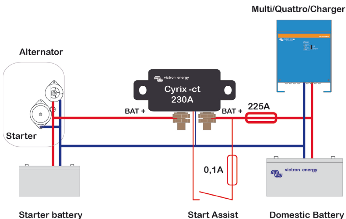
Cyrix-ct 12/24-230: schemat ideowy
