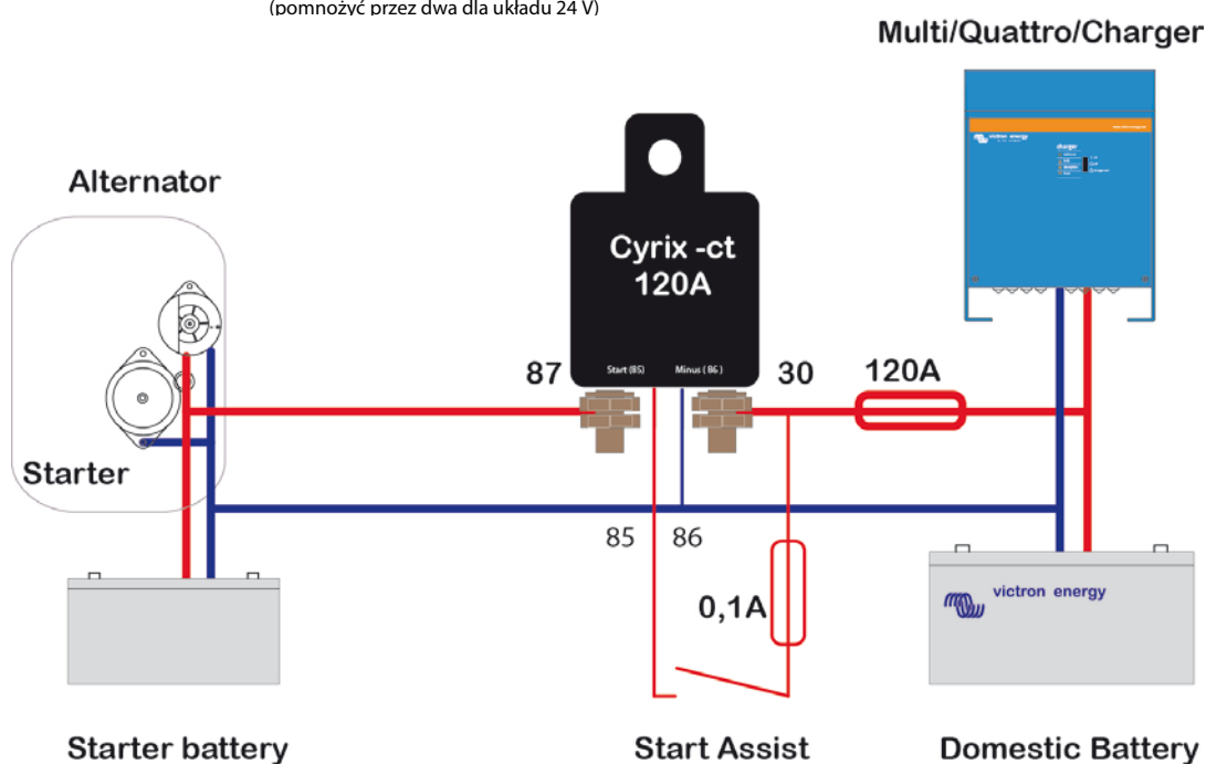
Cyrix-ct 12/24-120: schemat ideowy
