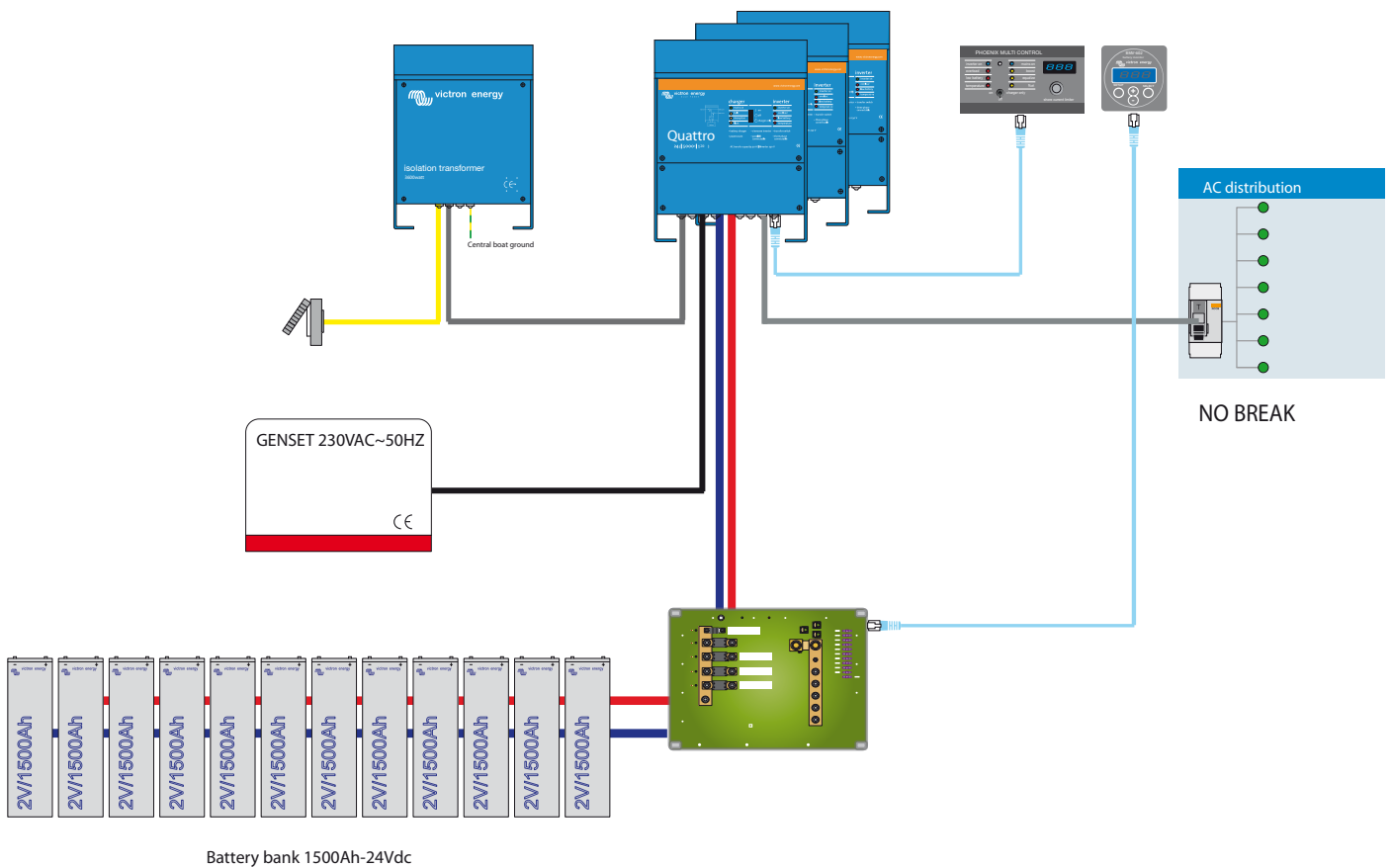
3 x 5Kw Quattro system
